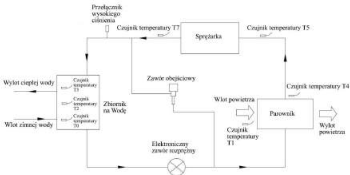
Rys. 1. Schemat poglądowy układu z zaworem obejściowym
