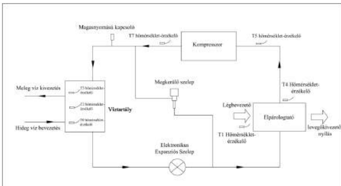
1. ábra A rendszer sematikus áttekintése megkerülő szeleppel
