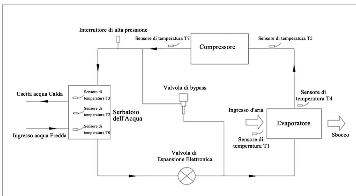
Fig. 1. Schema generale del sistema con valvola di bypass
