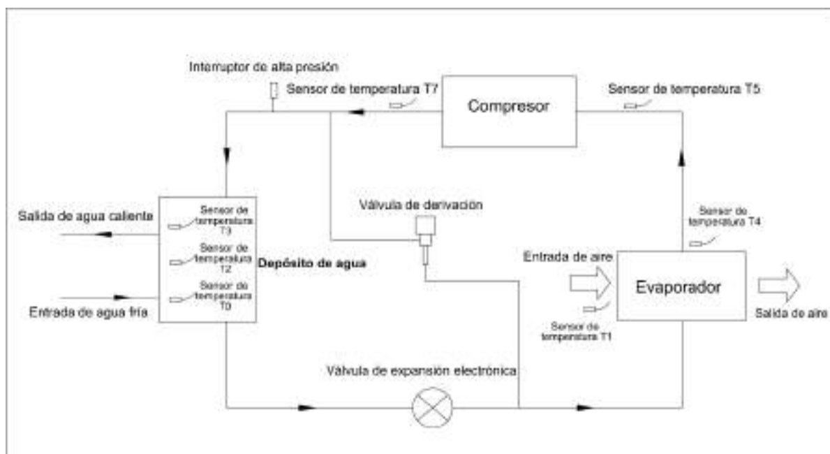
Fig. 1. Vista esquemática del sistema con válvula de derivación
